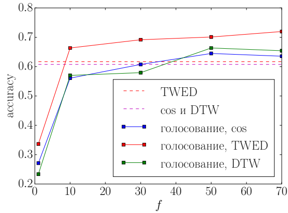
Рис. 13: Сравнение значений ассигасу для усреднения и голосования при различных значениях f .
