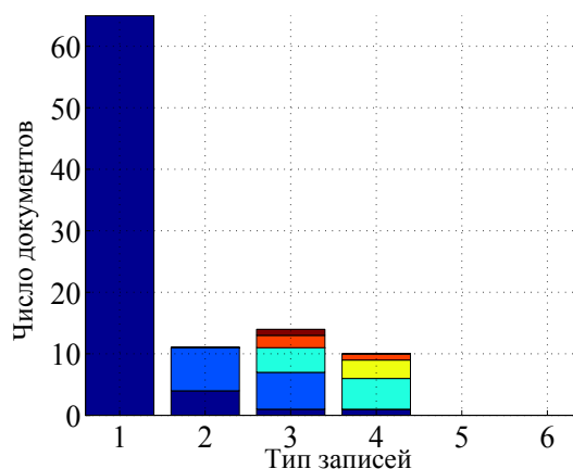
Рис. 16: Полученная кластеризация записей.
