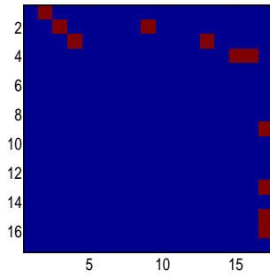
Рис. 5: Полученная матрица переходов \hat{\mathbf{Z}}_f .
