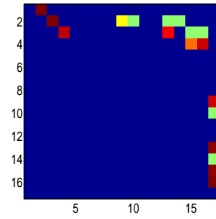
Рис. 4: Полученная матрица вероятности переходов \mathbf{P}_f .
