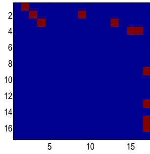
Рис. 3: Исходная матрица переходов \mathbf{Z}_f .
