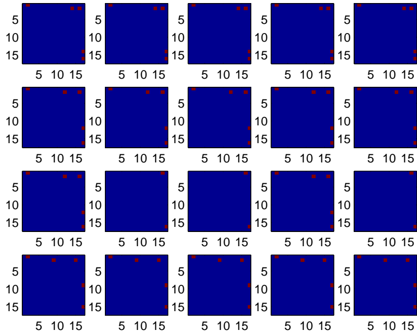
Рис. 7: Полученные матрицы переходов \mathbf{Z}_f .
