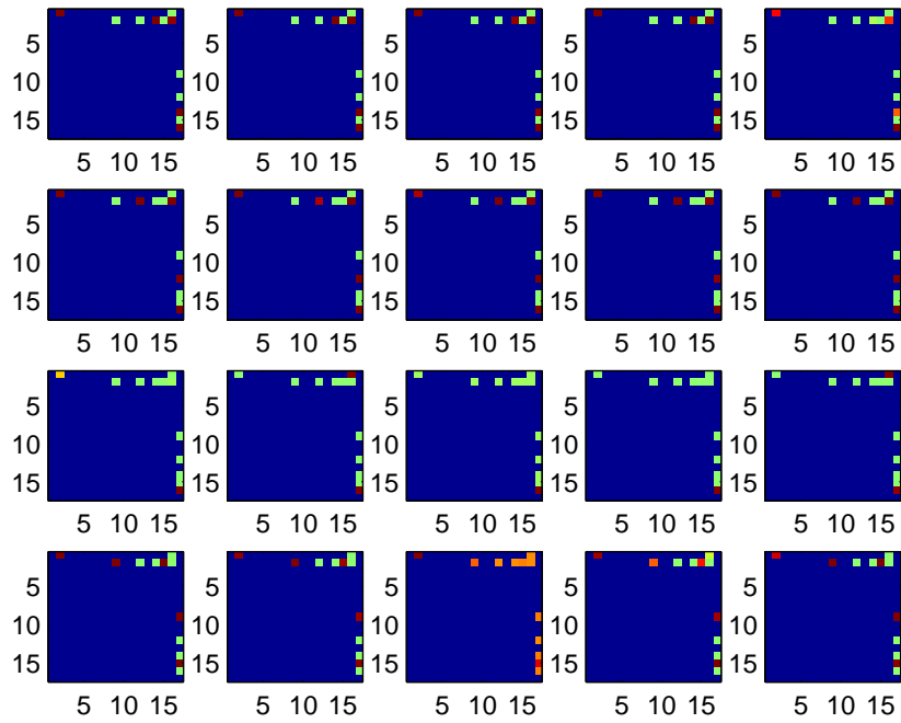
Рис. 6: Полученные матрицы вероятностей переходов \mathbf{P}_f .
