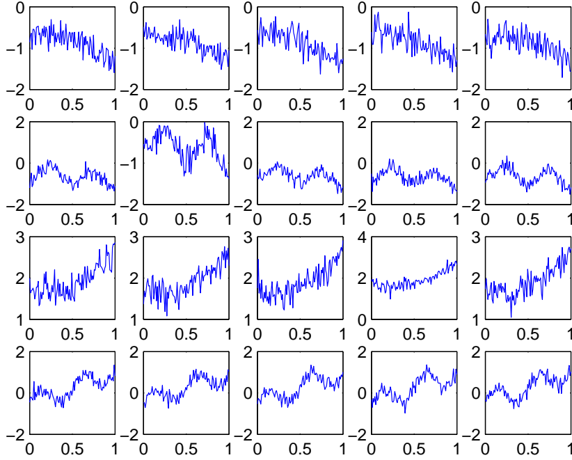
Рис. 2: Вид исходных данных.
